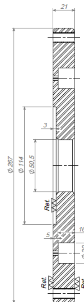
SEÇÃO A-A
